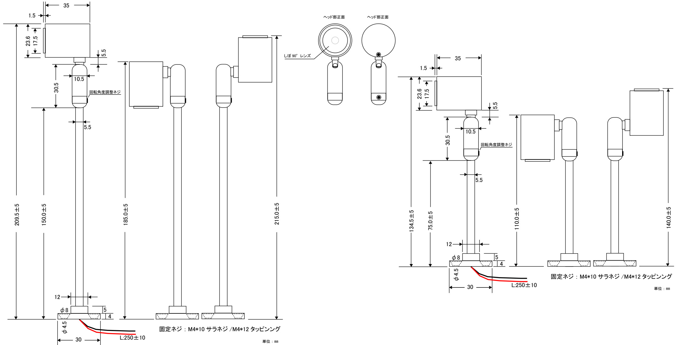
外形図: JCN-S-X001-CW-1W-150 / JCN-S-X001-WW-1W-150
